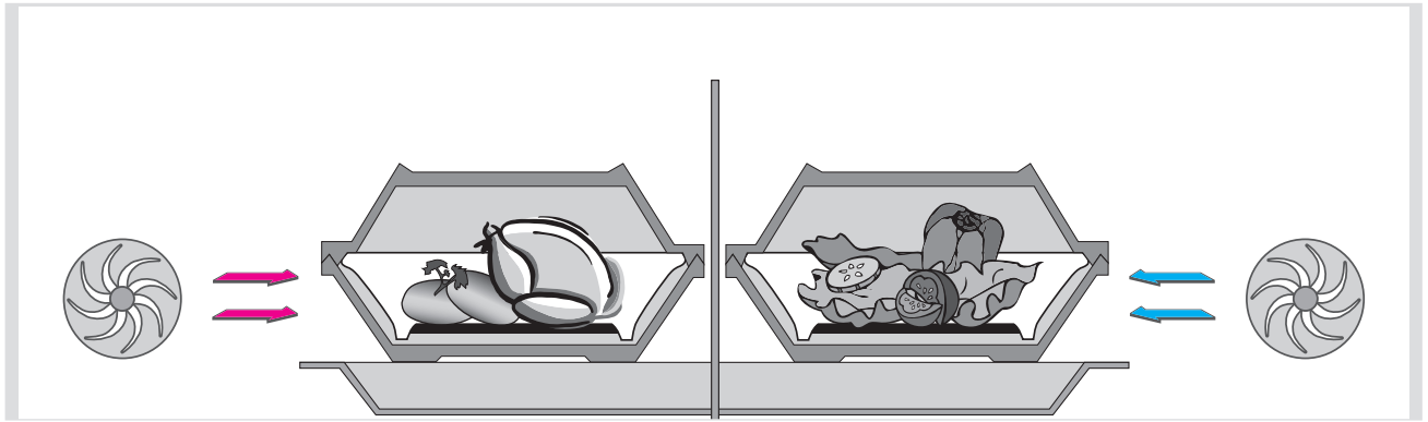
Heißluftgebläse (rot), Kaltluftgebläse (blau), portioniertes Tablett mit Klimateiler Hot air fan (red), cold air fan (blue), tray laid out in portions with temperature divider
